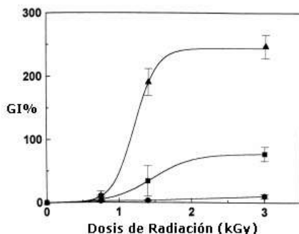
Figura 4.2 – Efecto de la dosis de radiación sobre el grado de injerto de fibras huecas de PE hidrofílicas inmersas en soluciones de 1% (●), 5% (■) y 10% (▲) de GMA en 50% metanol. Dosis total 3 kGy, fuente Gamma-cell ^{60}\text{Co} (adaptada de Grasselli y col. [6]).
