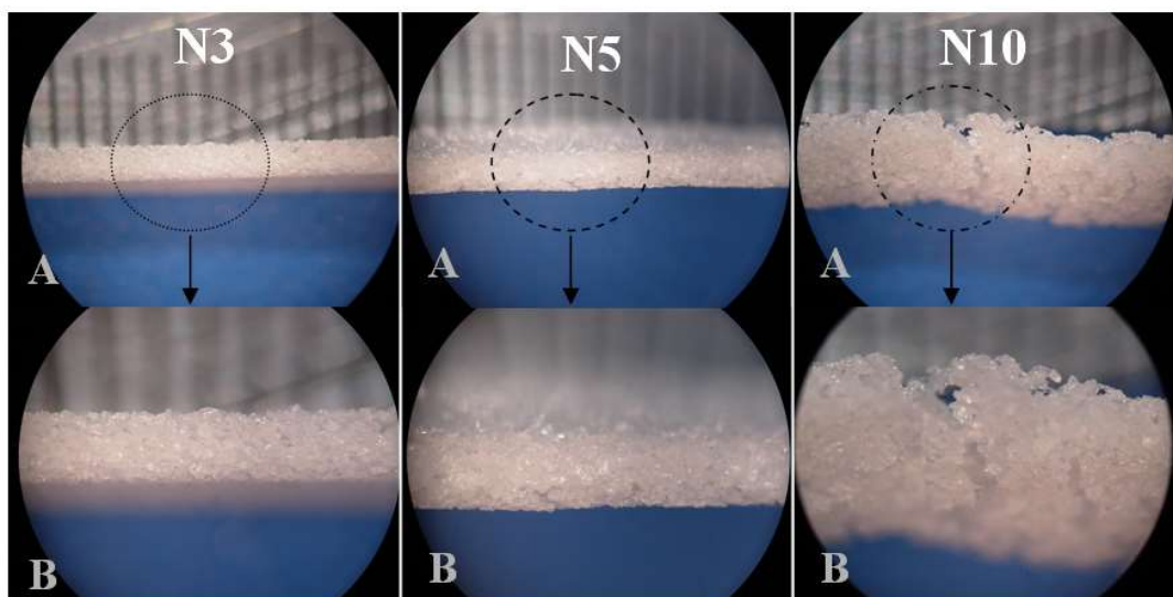
Figura 3.3 – Fotografías ampliadas de perfiles de PE poroso preirradiado en aire y copolimerizado con AAm: N3 (10% AAm, mezcla etanol agua), N5 (10% AAm, en agua) y N10 (20% AAm, en agua). Aumento 1,5x (A) y 3x (B) en lupa. En círculo: zona de A ampliada en B.
