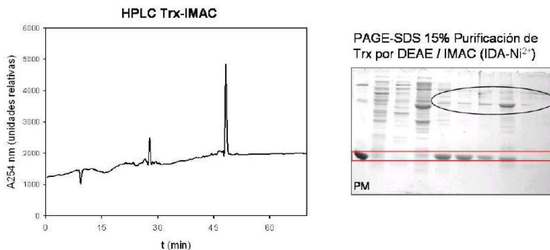
Figura B.3 – Análisis del proceso de purificación de rTrx en un solo paso a través de una IMAC ( \text{IDA-Ni}^{2+} ). Cromatograma HPLC-RP y PAGE-SDS 15 %, factor de pureza estimado >80 %. Se observa a la Trx (recuadro) y a las proteínas contaminantes que son separadas por la DEAE (óvalo).
