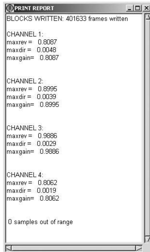
Figura 8.4: Ejemplo de impresión de reporte generado por Gtconvolve una vez que se procesaron los datos de entrada.
