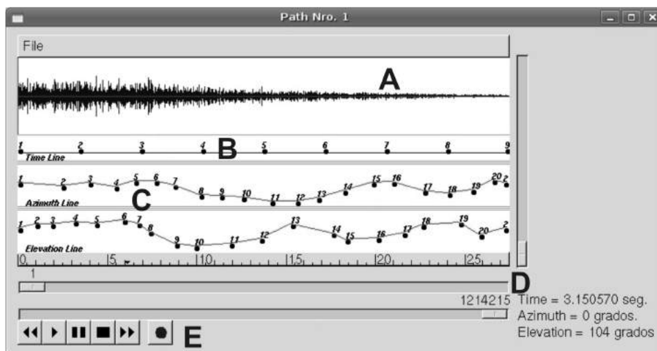
Figura 8.8: Audio File Window. Permite la visualización de los archivos relacionados con cada trayectoria, además de la coordinación temporal de los puntos, rotación en acimut y elevación. En algunas versiones se permite la reproducción del archivo de audio.
