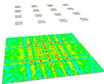
Figura 9.10: Diagrama de Radiación de la Disposición Cuadrícula – los colores indican un máximo Nivel de Presión Sonora (color rojo – 115 dBSPL), hasta un mínimo Nivel de Presión Sonora (40dBSPL) Diseño y simulación: Daniel Hernández
