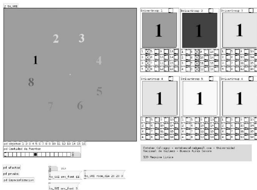
Figura 8.11: Pantalla principal de GUISPA. A la izquierda se puede apreciar el simulador de sala con 8 objetos rodeando un sweet spot; a la derecha los 6 módulos que permiten agrupar fuentes y moverlas de forma coordinada.
