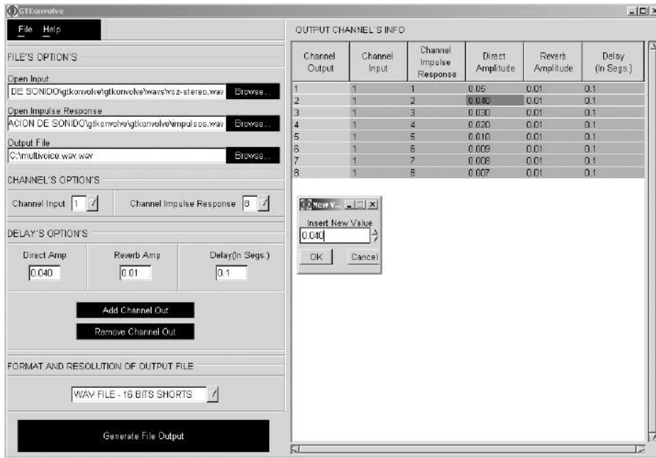
Figura 8.3: Ejemplo de cómo cambiar el valor de los casilleros previamente configurados.
