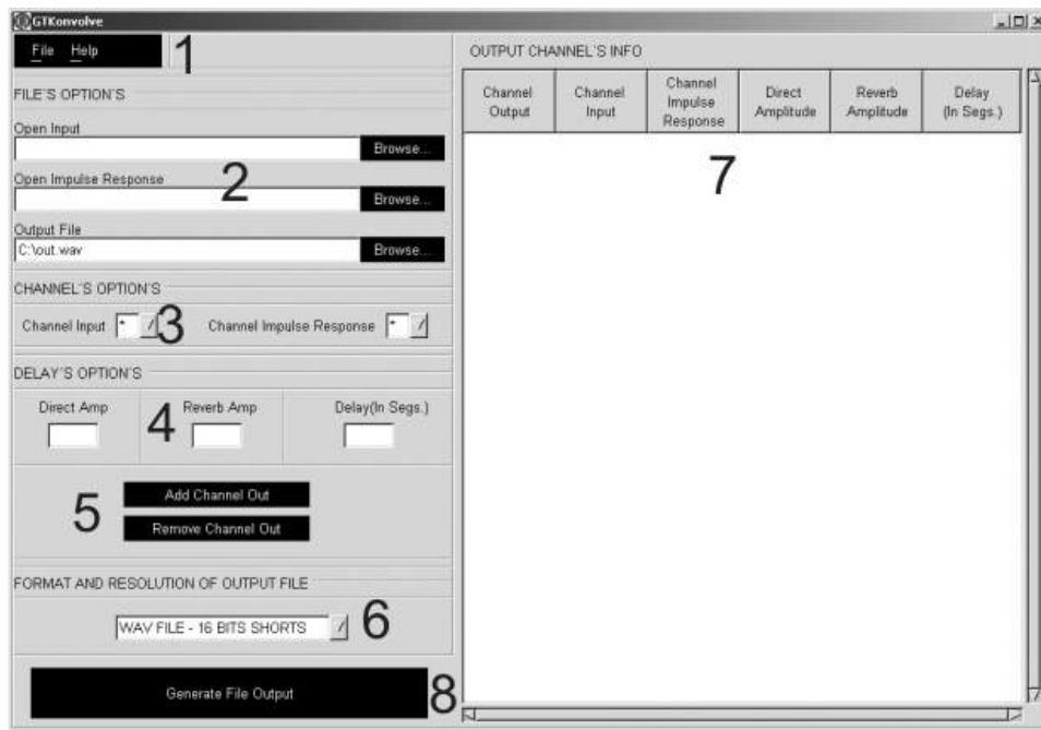
Figura 8.1: Frontend de Gtkonvolve. 1) Menú principal; 2) ingreso de la ruta del archivo de audio, respuesta a impulso y archivo de salida; 3) elección del canal del archivo de audio y el canal del archivo de las respuestas a impulso a combinar; 4) Configuración de la amplitud del sonido directo, de la reverberación y si se quiere agregar un delay entre ambos; 5) agregar o quitar combinaciones; 6) elección del formato y resolución del archivo de salida; 7) Información de las combinaciones de las que estará compuesto el archivo de salida; 8) Generación del archivo de salida
