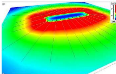
Figura 9.5: Patrón de radiación del sistema de reproducción de “Oí(r) el ruido” – Diseño: Daniel Hernández.
