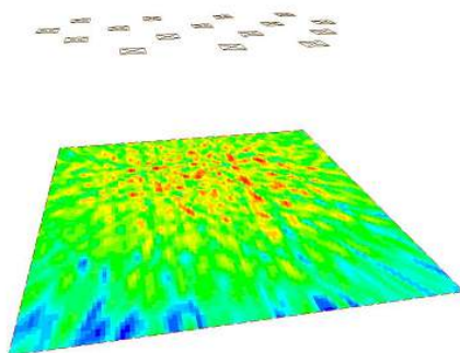
Figura 9.7: Diagrama de Radiación de la Disposición Hexágono Truncado – los colores indican un máximo Nivel de Presión Sonora (rojo – 115 dBSPL), hasta un mínimo Nivel de Presión Sonora (azul - 40dBSPL) Diseño y simulación: Daniel Hernández.
