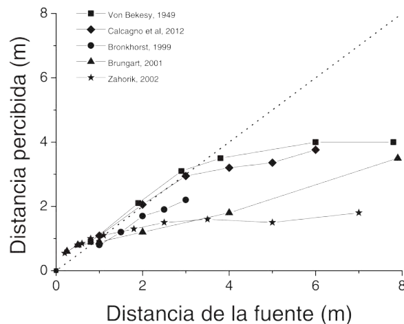
Figura 3.2: Diferentes curvas de PAD obtenidas de artículos que utilizan varios sistemas de medición. Es interesante observar como los trabajos realizados en entornos acústicos virtuales presentan un nivel de subestimación más marcado.
