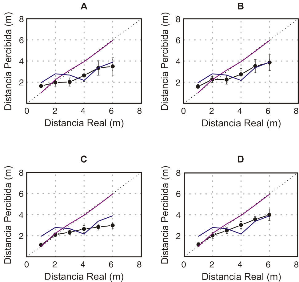
Figura 7.4: Ruido Rosa filtrado centrado en 500Hz con diferentes anchos de banda. (A)– 1/12 octava, n=8 : valor medio de los juicios de distancia como una función de la distancia real de la fuente sonora utilizando como estímulo ruido rosa centrado en 500Hz con un ancho de banda de 1/12 de octava; (B) – 1/6 octava, n=8 : valor medio de los juicios de distancia como una función de la distancia real de la fuente sonora utilizando como estímulo ruido rosa centrado en 500Hz con un ancho de banda de 1/6 de octava; (C)– Octava, n=8 : valor medio de los juicios de distancia como una función de la distancia real de la fuente sonora utilizando como estímulo ruido rosa centrado en 500Hz con un ancho de banda de una octava; (D)– Octava y Media, n=8 : valor medio de los juicios de distancia como una función de la distancia real de la fuente sonora utilizando como estímulo ruido rosa centrado en 500Hz con un ancho de banda de una octava y media. En todas las figuras se agregó para comparación la respuesta para ruido rosa (línea púrpura) y la respuesta para un tono de 500Hz (línea azul).
