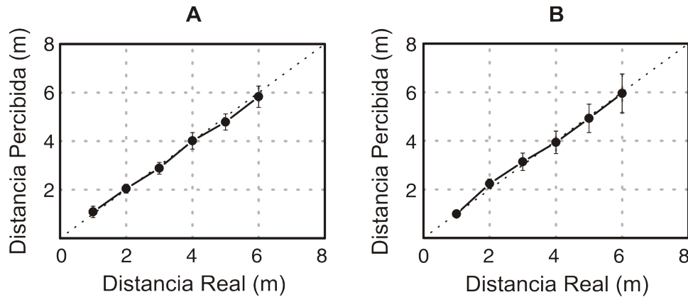
Figura 7.1: (A)- Ruido Blanco , n=8 : valor medio de los juicios de distancia como una función de la distancia real de la fuente sonora utilizando como estímulo ruido blanco; (B)- Ruido Rosa , n=8 : valor medio de los juicios de distancia como una función de la distancia real de la fuente sonora utilizando como estímulo ruido rosa.
