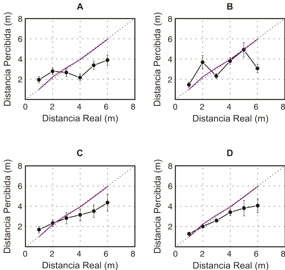
Figura 7.2: (A) – Tono 500Hz, n=8 : valor medio de los juicios de distancia como una función de la distancia real de la fuente sonora utilizando como estímulo un tono puro de 500Hz; (B) – Tono 1KHz, n=8 : valor medio de los juicios de distancia como una función de la distancia real de la fuente sonora utilizando como estímulo un tono puro de 1KHz;– (C), Tono 2KHz, n=8 : valor medio de los juicios de distancia como una función de la distancia real de la fuente sonora utilizando como estímulo un tono puro de 2KHz; (D)– Tono 4KHz, n=8 : valor medio de los juicios de distancia como una función de la distancia real de la fuente sonora utilizando como estímulo un tono puro de 4KHz; En todas las figuras se agregó para comparación la respuesta obtenida con ruido rosa en el experimento 1 (línea púrpura).
