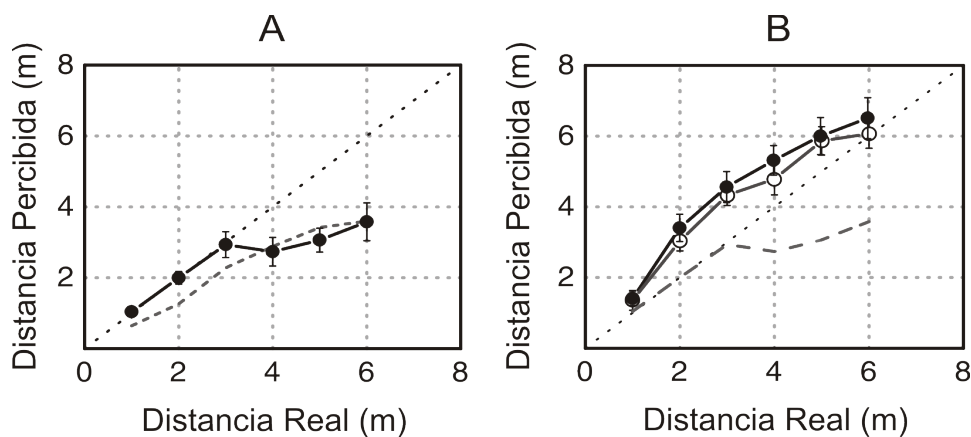
Figura 6.4: Experimento 2 – grupo A: Percepción Auditiva de Distancia (sin conocimiento previo de la sala). (A) Valor medio de los juicios de distancia como una función de la distancia real obtenida sin pistas visuales (condición 1, n=8 , círculos negros). Como referencia se agregó, mediante una línea gris discontinua, los resultados obtenidos en el experimento 1 (condición i para visión). (B) Valor medio de los juicios de distancia como una función de la distancia real obtenida con dos (condición ii, n=8 , círculos blancos) y cuatro pistas visuales (condición i, para percepción auditiva de distancia).
