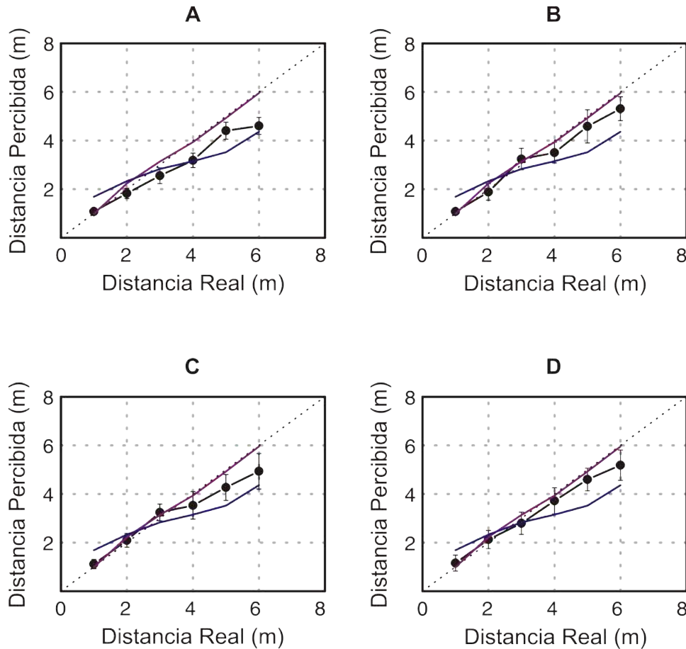
Figura 7.6: Ruido Rosa filtrado centrado en 2KHz con diferentes anchos de banda. (A)– 1/12 octava n=8 : valor medio de los juicios de distancia como una función de la distancia real de la fuente sonora utilizando como estímulo ruido rosa centrado en 2KHz con un ancho de banda de 1/12 de octava; (B)– 1/6 octava n=8 : valor medio de los juicios de distancia como una función de la distancia real de la fuente sonora utilizando como estímulo ruido rosa centrado en 2KHz con un ancho de banda de 1/6 de octava; (C) – Octava, n=8 : valor medio de los juicios de distancia como una función de la distancia real de la fuente sonora utilizando como estímulo ruido rosa centrado en 2KHz con un ancho de banda de una octava; (D) – Octava y Media, n=8 : valor medio de los juicios de distancia como una función de la distancia real de la fuente sonora utilizando como estímulo ruido rosa centrado en 2KHz con un ancho de banda de una octava y media. En todas las figuras se agregó para comparación la respuesta para ruido rosa (línea púrpura) y la respuesta para un tono de 2KHz (línea azul).
