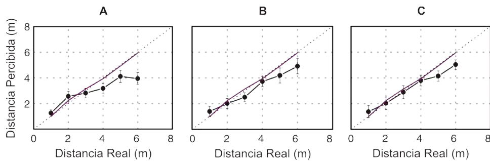
Figura 7.3: (A) – 20Hz-1KHz, n=8 : valor medio de los juicios de distancia como una función de la distancia real de la fuente sonora utilizando como estímulo ruido rosa filtrado entre 20Hz y 1KHz; (B) -1KHz-3KHz, n=8 : valor medio de los juicios de distancia como una función de la distancia real de la fuente sonora utilizando como estímulo ruido rosa filtrado entre 1KHz y 3KHz; (C)– 3KHz-20KHz, n=8 : valor medio de los juicios de distancia como una función de la distancia real de la fuente sonora utilizando como estímulo ruido rosa filtrado entre 3KHz y 20KHz; En todas las figuras se agregó para comparación la respuesta obtenida con ruido rosa en el experimento 1 (línea purpura).
