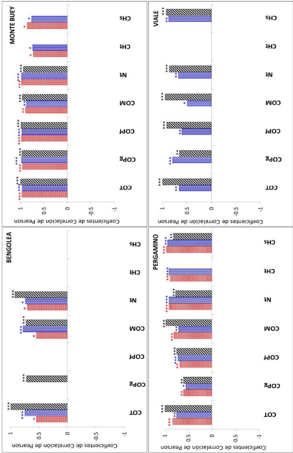
Figura 4.4: Análisis de correlación de pearson en los cuatro ambientes estudiados, del COT y sus fracciones: COPg, COPf, COM, del Nt y de los CHs y CHt con: el COT, la fracción fácilmente extraíble de glomulina (GRSP-FE), y la fracción total de glomulina (GRSP-Total). Los asteriscos sobre las columnas representan los p-valores significativos: * p < 0.05, ** p < 0.01, *** p < 0.001. Cuando los p-valores fueron no significativos (p>0.05) la correlación se consideró nula.
