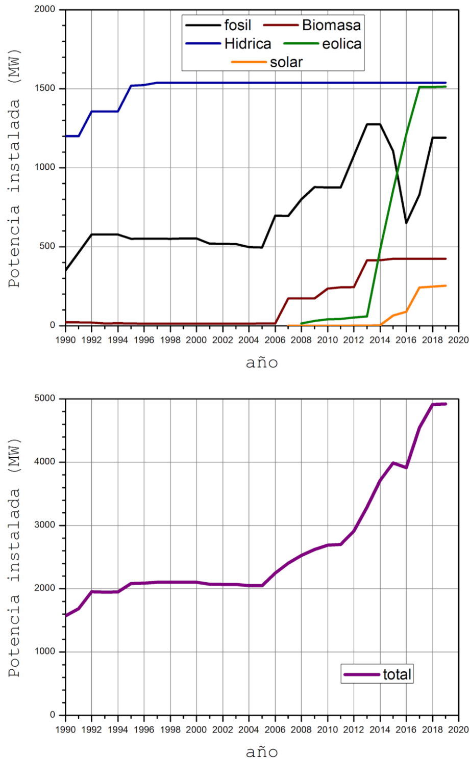
Figura 2: Potencia instalada por fuente (arriba) y total (abajo) 1990-2019. Fuente: elaboración propia en base a datos de MIEM-Datos abiertos (2021).
