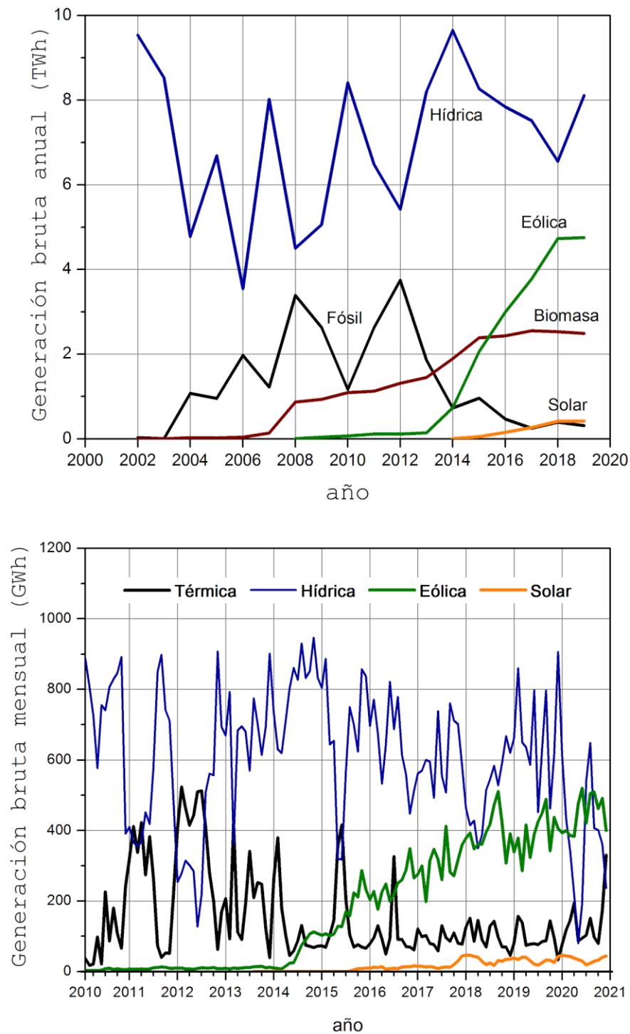
Figura 3: Generación bruta anual 2000-2019 por fuente (arriba). Generación bruta mensual 2010-2021 por fuente (abajo). En este último gráfico la energía de generación térmica abarca a la fósil y a la biomasa. Fuente: elaboración propia en base a datos de MIEM-Datos abiertos (2021).
