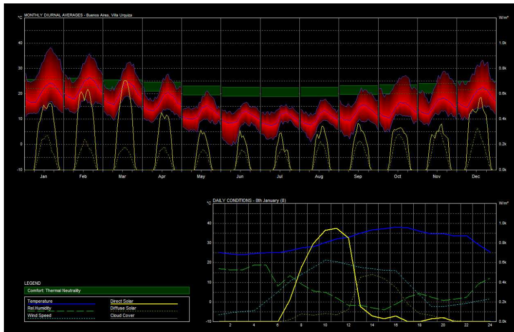
Figura 5: En la herramienta Ecotect Analysis - Weather Tool, con archivos de clima de la ciudad de Buenos Aires, la gráfica muestra promedios mensuales de temperatura en °C e incidencia de irradiancia solar W/m 2 en superficies. Asimismo se define una franja de confort térmico para todo el año. Se visualizan mayormente entre noviembre y marzo temperaturas por encima de la zona de confort con altos valores de radiación directa
