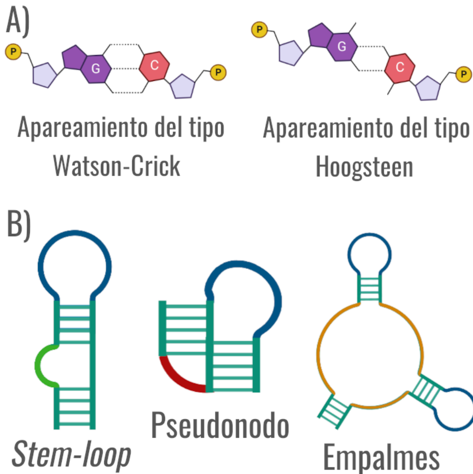
Figura II.2: Representación pictórica de apareamientos y estructuras secundarias típicas de los ARN. Panel A: Representación de los apareamientos del tipo Watson-Crick y Hoogsteen entre una Guanósina (color violeta) y una Citosina (color naranja). Los puentes de Hidrógeno entre ambas moléculas se representan con líneas punteadas Panel B: Representación pictórica para las estructuras secundarias de un stem-loop , un pseudonodo, y un empalme de tres vías. Las regiones apareadas se representan en verde, mientras las regiones de simple cadena correspondientes a loops , burbujas, uniones de pseudonodos y empalmes se representan en azul, verde claro, rojo y amarillo, respectivamente.
