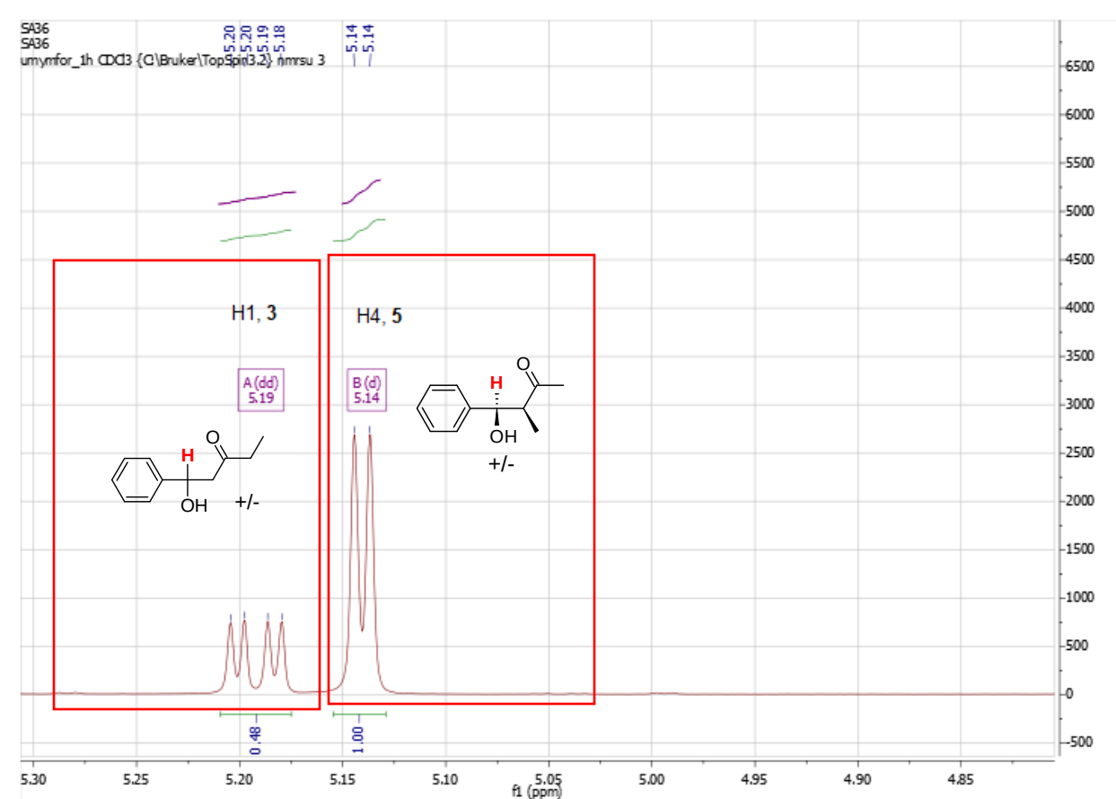
Figura 3. Región del espectro RMN- 1 H de la mezcla de cetos 3 y 5. Se resaltan las señales correspondientes al hidrógeno del carbono 1 del cetol 3 y al hidrógeno del carbono 4 del cetol 5, utilizadas para calcular la proporción de los cetos de dicha muestra.
