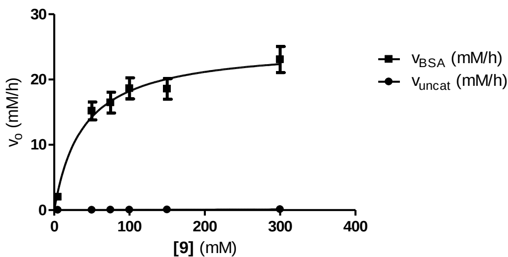
Figura 6. Velocidad inicial ( v_0 ) versus concentración de p -nitrobenzaldehído ( [9] ) para la condensación aldólica catalizada por BSA de 9 y ciclohexanona 5 M en etanol a 45 °C y 200 rpm. Las conversiones fueron determinadas por absorción a 330 nm en un lector de placas Cytation 5 (ver sección 3.2.12).
