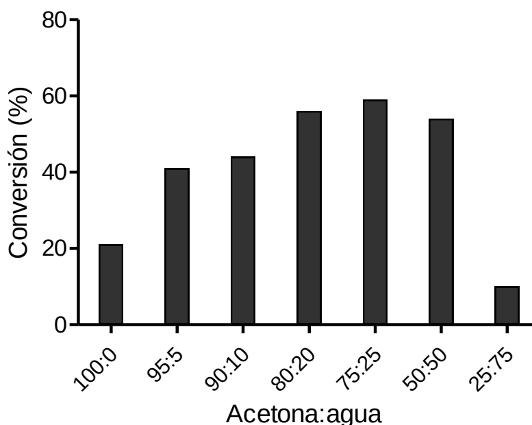
Figura 2. Efecto del contenido de agua en la formación de benzalacetona ( 3a ) a 30°C con 27 mg de BSA (sección 2.2.2). Valores de conversión a 120 h de reacción, determinados por HPLC.
