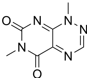
Figura 5. Estructura química de la toxoflavina
