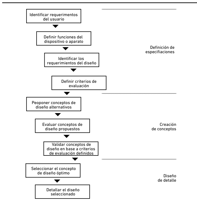
Figura 1. Esquema de método de diseño tecnológico estándar.
