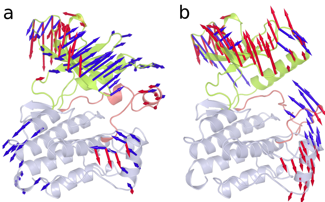
Figure 6.8: Modos SVD representativos U_1^1 (rojo) y U_1^2 (azul). En violeta, el lóbulo C, en verde, el lóbulo N y en rojo, el activation loop . Conforméromos inactivos (a) y activos (b).
