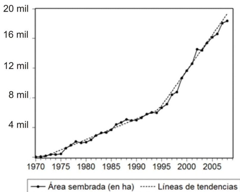
Gráfico 3. Área sembrada con soja (1970-2007) y líneas de tendencia
