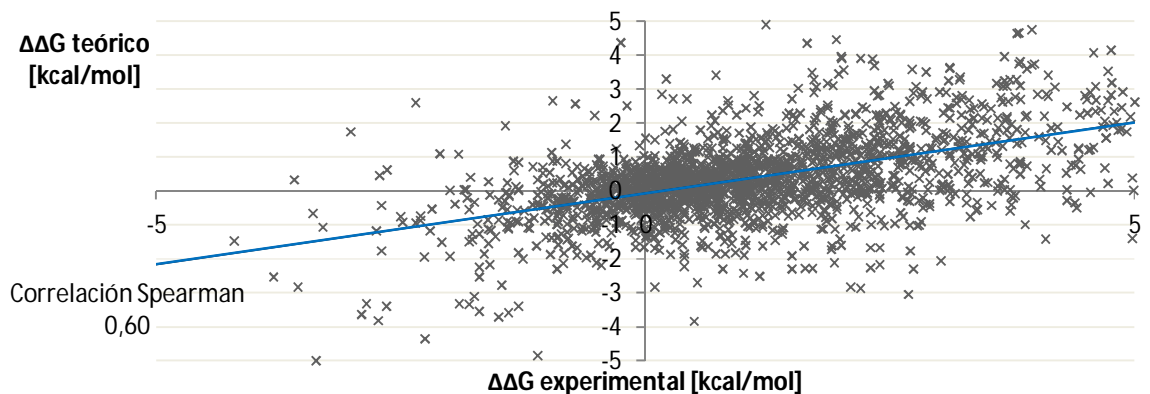
Figura 29. Correlaciones obtenidas por los métodos (a) I-Mutant, (b) Fold-X y (c) D-Mutant, utilizando todos los conforméros disponibles derivados de la PCDB.
