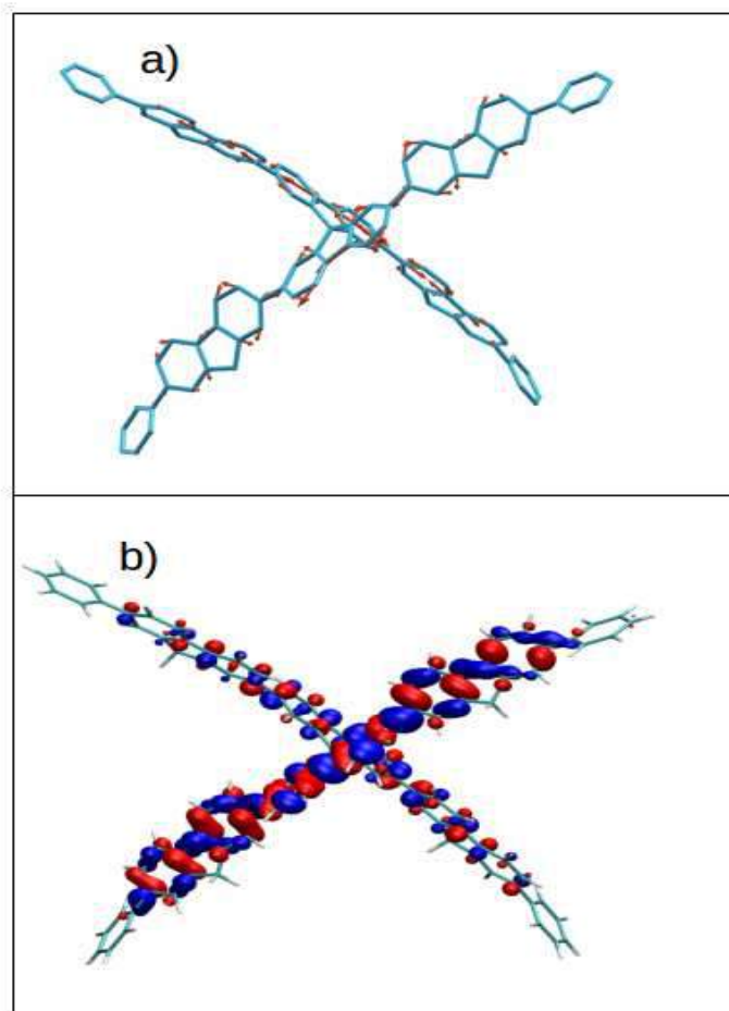
Figura 4.4: a-) Vector de acoplamiento no-adiabático para una trayectoria específica a 10K en el tiempo efectivo de la transición S_2 \rightarrow S_1 . b-) Localización de la densidad de transición electrónica en el tiempo efectivo de la transición S_2 \rightarrow S_1 .
