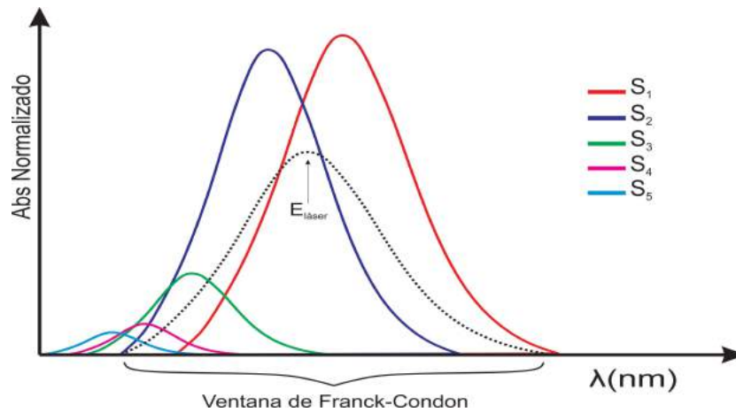
Figura 3.3: Representación de la ventana de Franck-Condon para seleccionar el estado electrónico excitado inicial.
