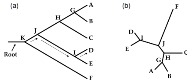
Figura 1.3. Estructura de un árbol filogenético con raíz (a) y un árbol filogenético sin raíz (b). Los dos árboles tienen la misma topología. Un árbol con raíz generalmente se dibuja con la raíz a la izquierda. Las letras A, B, C, D, E y F representan los nodos externos o OTUs. Las letras G, H, I, J y K representan los nodos internos o HTUs, donde la K es el nodo raíz. El árbol raíz carece de este nodo raíz ( root ). Las líneas entre cada nodo son las ramas. En el árbol con raíz, la flecha indica la dirección del proceso evolutivo (por ejemplo, desde el nodo raíz K hasta el nodo externo D). En el árbol sin raíz, por el contrario, la dirección del proceso evolutivo es desconocida.
