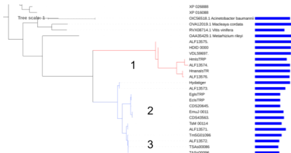
Figura 3.16 Árbol filogenético conteniendo los homólogos cercanos a EglSTRP mostrando en forma de barras los scores de rigidez (barras azules). Este score es el promedio de posiciones rígidas por proteína considerando como corte una probabilidad > 0.8. Cuanto menor es el score mayor es la flexibilidad de la proteína. Los números (1, 2 y 3) indican los nodos ancestrales comunes a 3 grupos principales de organismos: 1 corresponde al cluster de Hymenolepis , 2 al de Echinococcus y el 3 al de Taenia .
