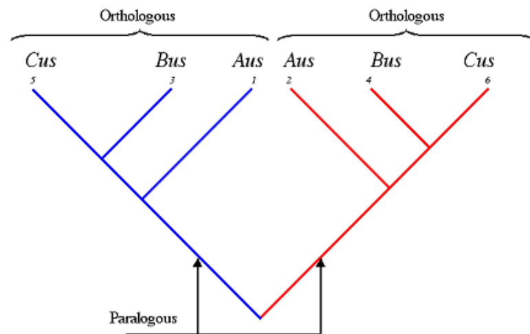
Figura 1.1. Evolución de genes ortólogos y parálogos.
