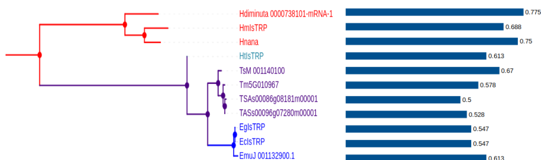
Figura 3.18. Árbol filogenético de las tiorredoxinas, reducido a EglSTRP y sus homólogas cercanas. En rojo, la familia Hymenolepididae , en violeta la familia Taeniidae y en azul el género Echinococcus . En cian se encuentra marcada la proteína de H. taeniaeformis , que es la más cercana a la familia Hymenolepididae .
