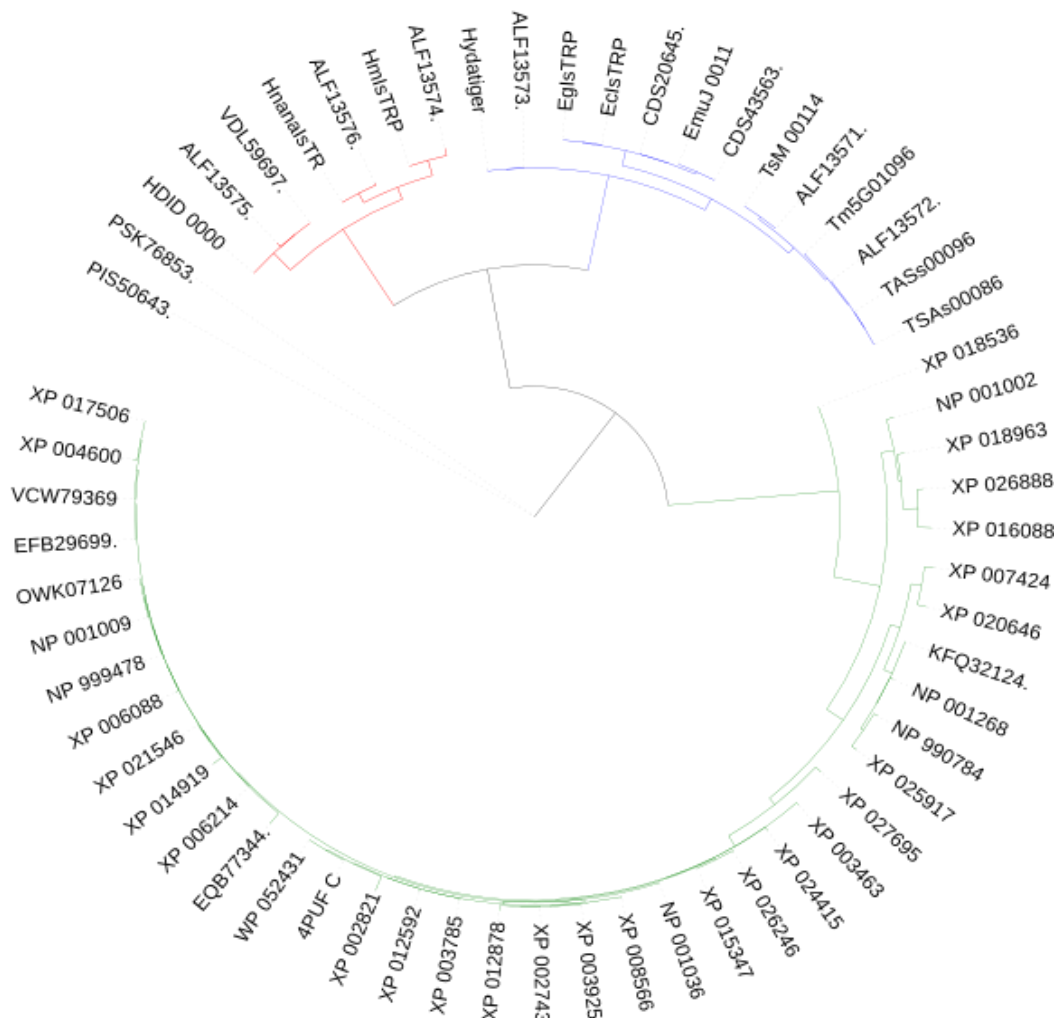
Figura 3.5 Estimación filogenética para las secuencias conteniendo las proteínas cercanas evolutivamente a Egl1sTRP así como las muy alejadas evolutivamente. El cluster rojo y azul contienen las secuencias cercanas a Egl1sTRP. Egl1sTRP se encuentra en el cluster azul que corresponde a organismos de la Familia Taeniidae mientras que las proteínas homólogas cercanas se encuentran en el cluster rojo conteniendo proteínas de la Familia Hymenolepididae . El cluster verde, claramente diferenciado de los dos anteriores contiene tioredoxinas canónicas de diversos organismos mayoremente vertebrados.
