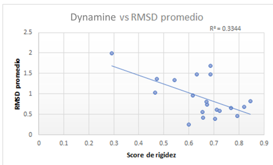
Figura 3.15 Correlación entre tiorredoxinas con diversidad conformacional conocida (RMSD promedio entre los cónformeros) y score de rigidez estimado usando el programa Dynamine
