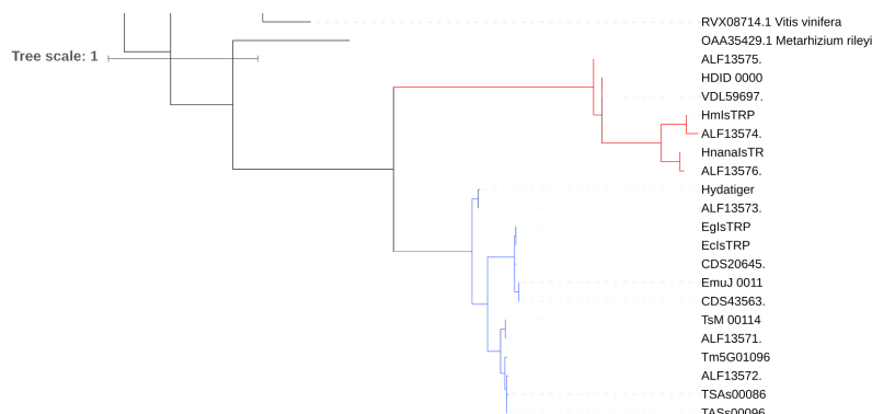
Figura 3.14 Árbol filogenético de las secuencias homólogas cercanas a EglSTRP. En el cluster azul se encuentra la EglSTRP (códigos: EglSTRP y EclSTRP) junto con secuencias del género Taenia , mientras que el cluster rojo contiene secuencias del género Hymenolepis .
