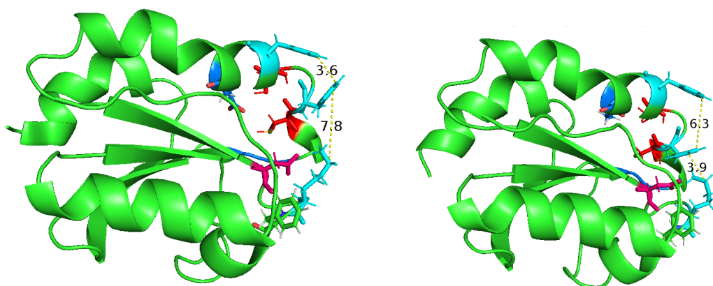
Figura 3.10 conformaciones alternativas de la EglSTRP. Estas conformaciones se pueden describir en función de 3 residuos: Phe 35, Phe 39 y Lys 63 (en cian). En la figura de la izquierda se aprecia que la Phe 35 establece una interacción pi-pi con la Phe 39 (distancia mínima registrada 3.6 Å), mientras que en la otra conformación (imagen de la derecha) la Phe 35 establece una interacción pi-catión con la Lys 63. En rojo se destacan las Cys del sitio activo.
