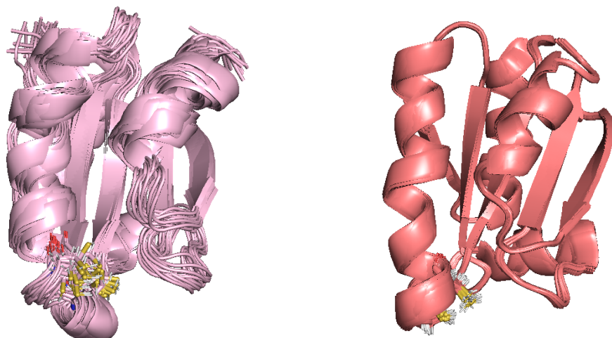
Figura 3.9 A la izquierda se muestra los 20 confórmers correspondientes a la EglSTRP destacando la presencia de las Cys del sitio activo. Para su comparación, a la derecha se muestran 40 confórmers correspondientes a la tiorredoxina humana en su estado reducido (PDB 1TRV).
