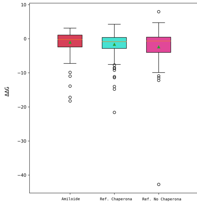
Figura 2.4. Distribución de los valores de ddG de distintas poblaciones. Cada columna contiene la información de los valores de ddG para todas las mutaciones ocurridas desde el ancestro raíz al ser humano. (Amiloide: proteínas amiloidogénicas; Ref. Chaperona: proteínas de referencia que interaccionan con chaperonas; Ref. No Chaperona: proteínas de referencia que no interaccionan con chaperonas). No se observan diferencias entre las distribuciones de amiloides y proteínas que interaccionan con chaperonas (p-value: 0.321), pero sí entre cada una de estas dos y las proteínas que no interaccionan con chaperonas (p-value: 0.0058 y 0.012, respectivamente).
