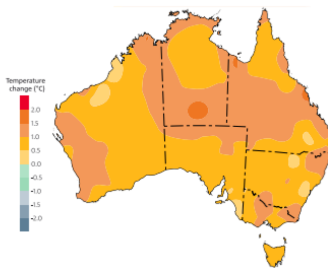
Figura 8. Variación en el clima de Australia (cambio de temperatura promedio en ^{\circ}\text{C} ) entre 1910 y 2013
